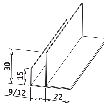
Γωνία περιμετρική «F» 15 x 34 x 3000mm
