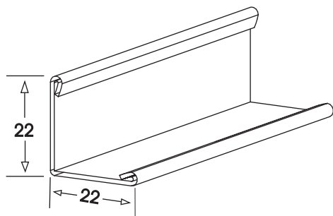
Γωνία περιμετρική «L» 22 x 22 x 3000mm
