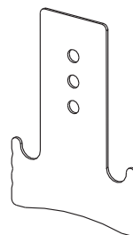
Άγκιστρο καναλιού ΚΩΔ.: AK 65
